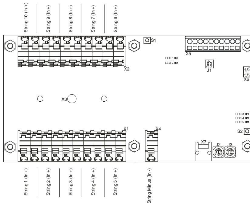
Abb. 5 Eingangsanschluss im KSM-Monitoring System
