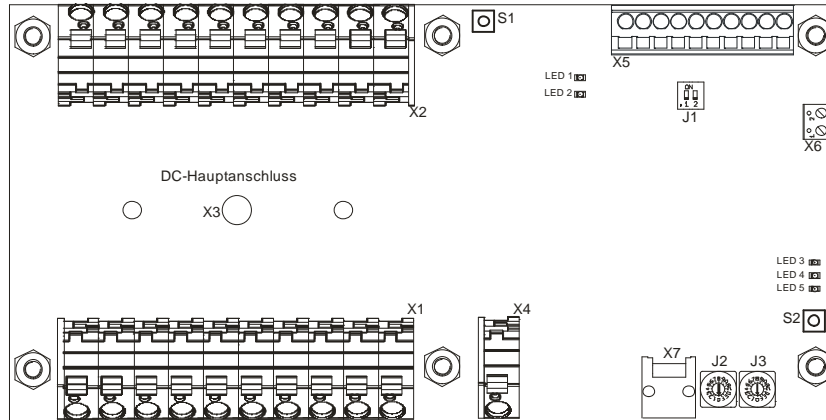
Abb. 6 Hauptleitungsanschluss im KSM-Monitoring System
