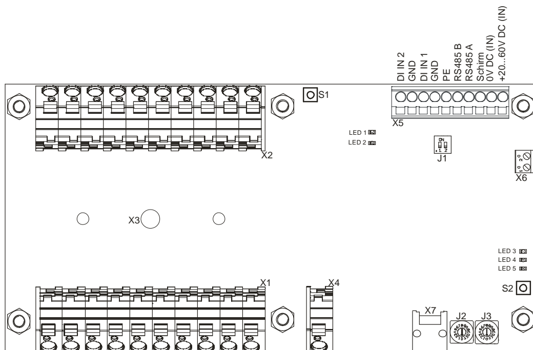
Abb. 3 Kommunikationsanschluss im KSM-Monitoring System
