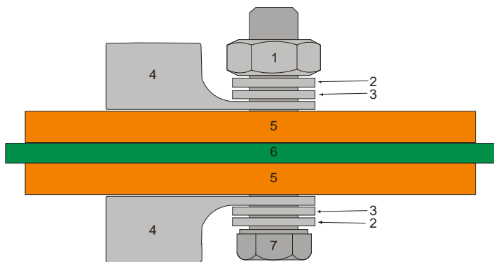
Abb. 7 Aufbau Befestigungspunkt Hauptleitungsanschluss
