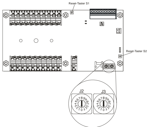
Abb. 9 Adresskodierschalter des KSM-Monitoring Systems
