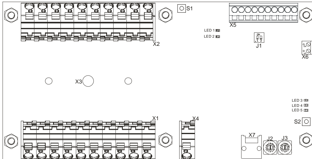
Abb. 1 Beispielaufbau des KSM-Monitoring System
