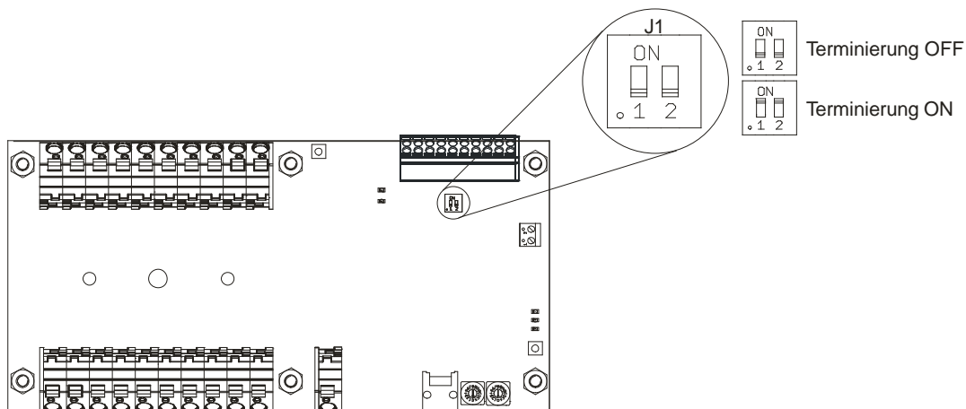
Abb. 8 Terminierung des KSM-Monitoring Systems
