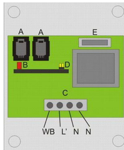
Abbildung 1 Anschl sse
